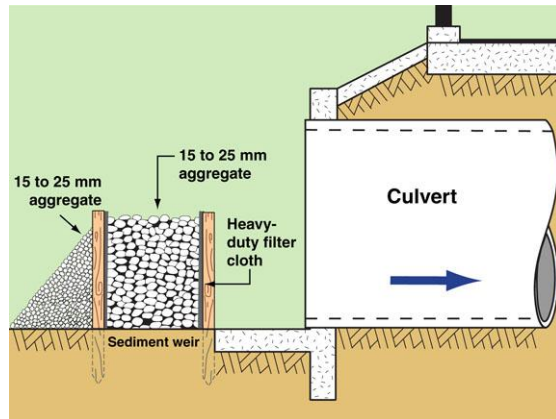
Sediment weir
