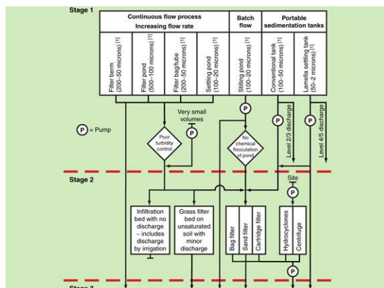
Site de-watering (Qld)
