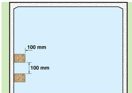
Longitudinal baffles
