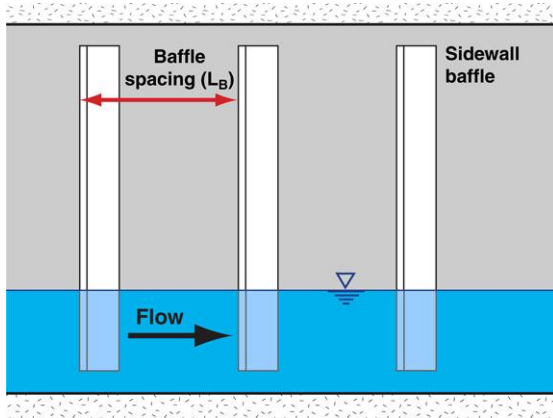
Baffle spacing
