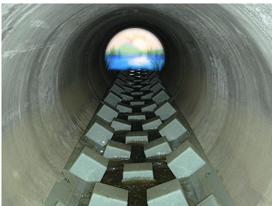
Spoiler baffles
