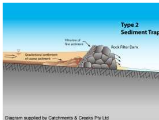
Type 2 sediment trap
